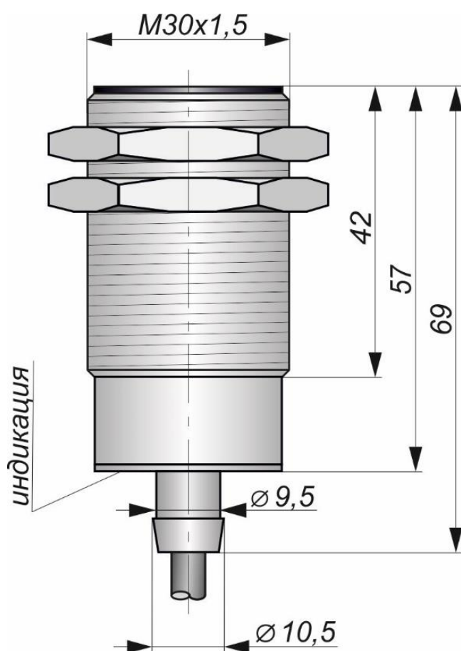
Габаритный чертеж
